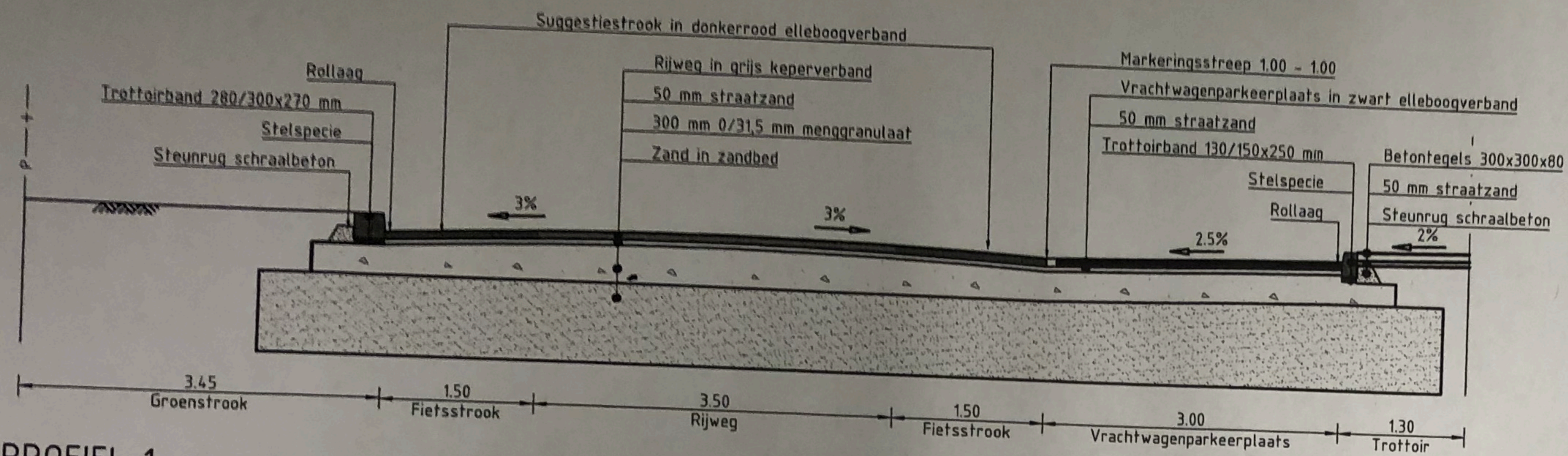
DWARSPROFIEL 1 SCHAAL 1:50
